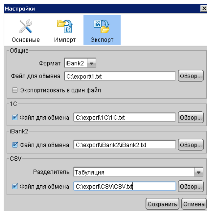
Рис. 3. Окно Настройки
